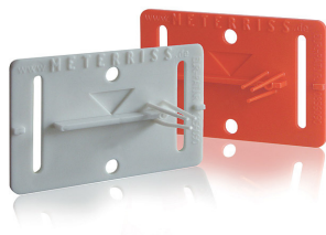
RS21 Meterriss-Plakette, selbstklebend zur dauerhaften Sicherung des Meterrisses bis nach den Putzarbeiten CHF 2.65* / Stück
