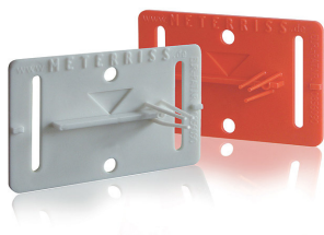
RS20 Meterriss-Plakette, zur dauerhaften Sicherung des Meterrisses bis nach den Putzarbeiten CHF 2.45* / Stück
